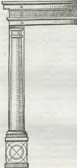
Tuſcana integra columnatio cum trabecatione.
